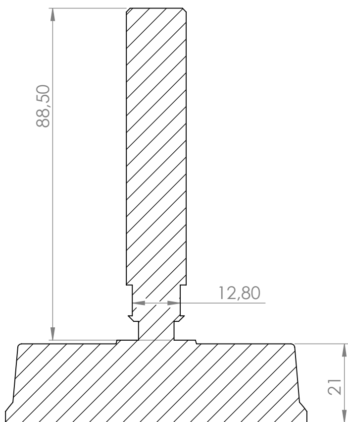
KESIT A-A
